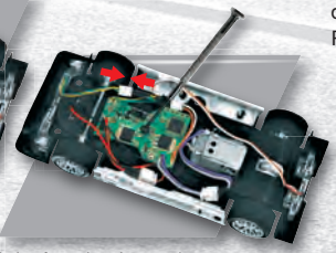
Platine festschrauben und Chassis schließen
