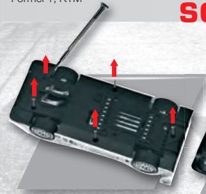
Schrauben lösen, Chassis abnehmen
